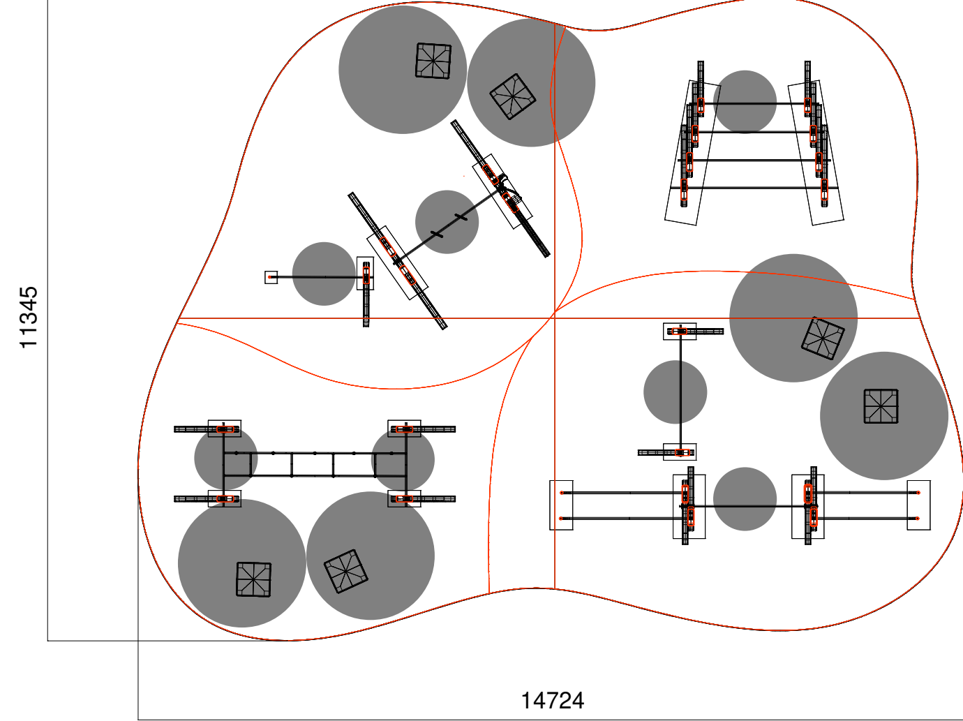
Obr. 53 - prostor vymezený pro cvičení určený normou ČSN EN 16630
